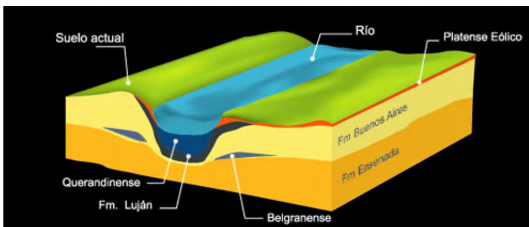
Figura 15: Esquema de formaciones pospampeana y pampeana
