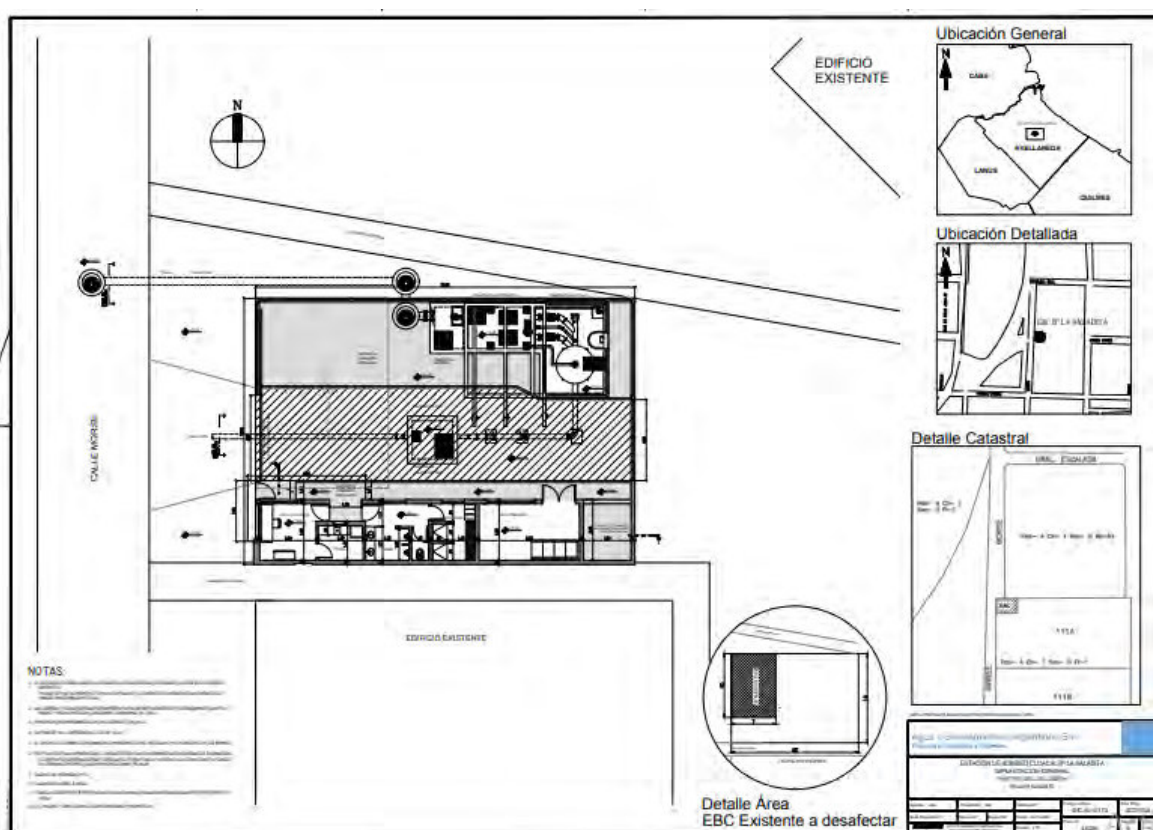
Figura 3: Implantación general de EBC B° La Saladita (SC70104)
